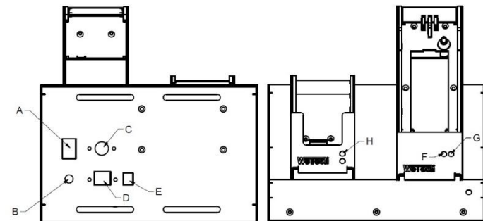
Schemazeichnung DC623BNC-695
